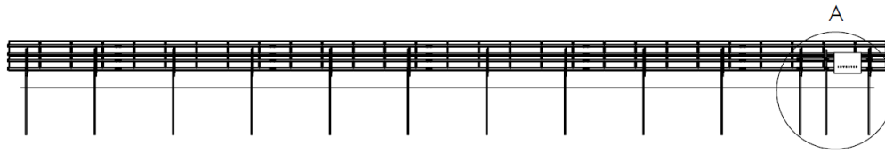
Figura 3. Desen orientativ – Detalii structurale – soluție pentru structura de montare a invertorului
