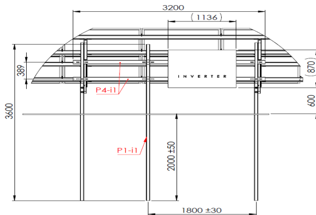
Figura 3. Desen orientativ – Detalii structurale – soluție pentru structura de montare a invertorului
